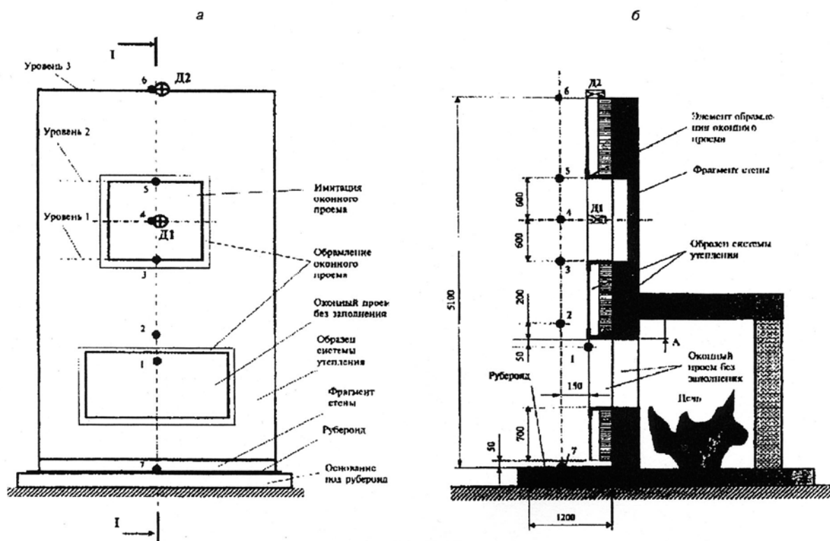
Рис. 1. Схема установки для огневых испытаний с образцом системы утепления:
