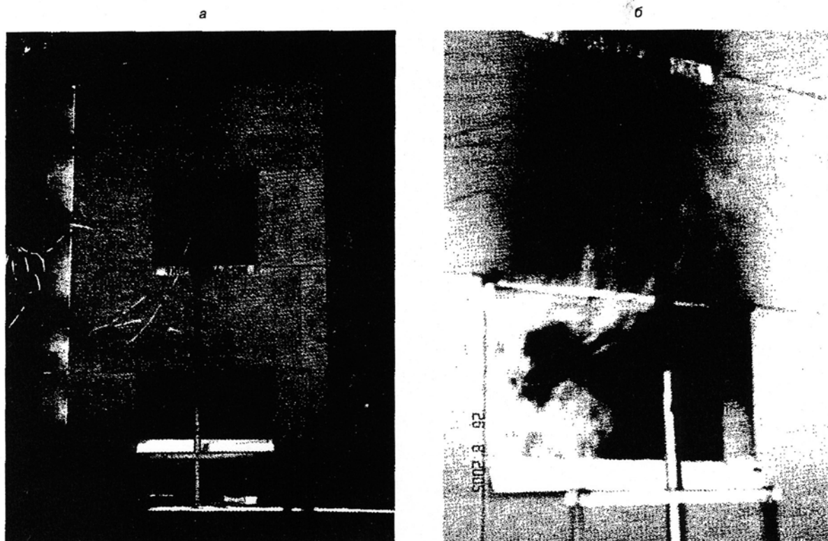
Рис. 2. Установка для огневых испытаний с образцом навесной фасадной системы «ФиброФасад»:
