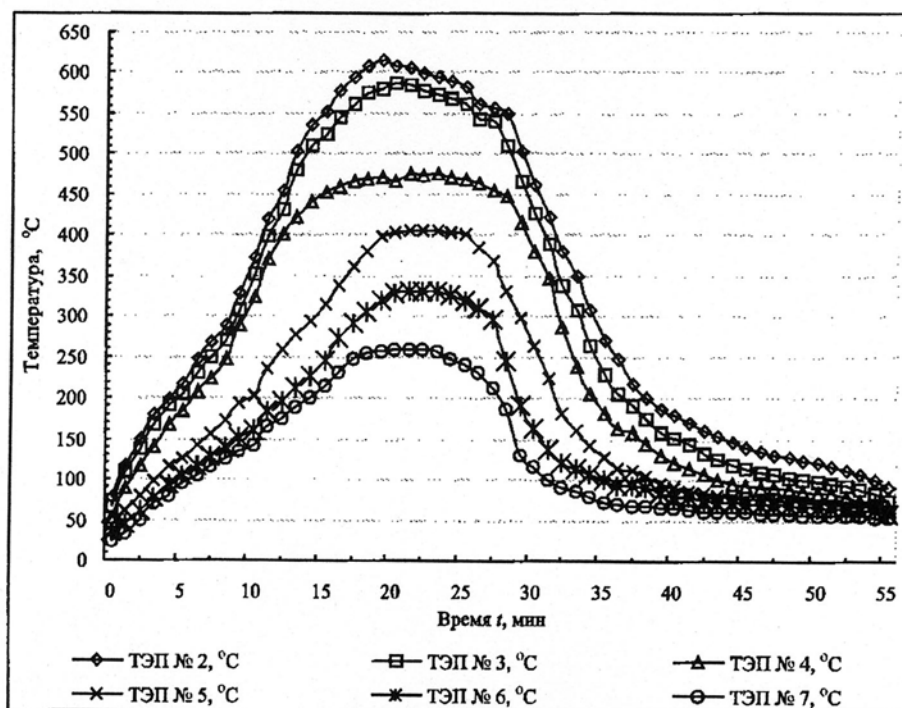
Рис. 4. Изменение в зависимости от времени температуры нагрева по высоте газовой колонки с внешней стороны образца фасадной системы в точках 2–7 (ТЭП № 2–7) на расстоянии 150 мм от лицевой поверхности образца
