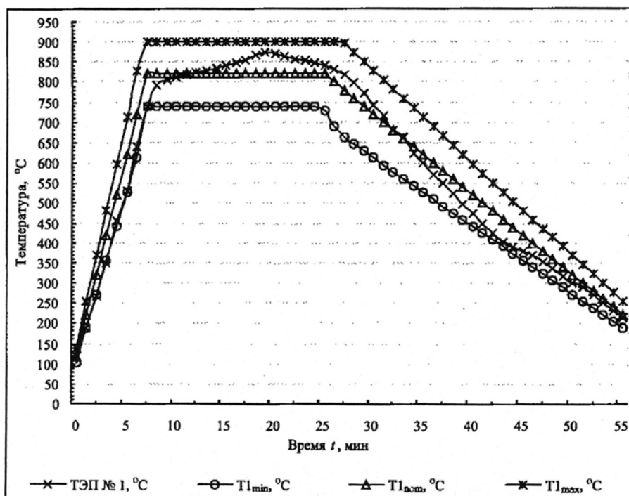
Рис. 3. Изменение в зависимости от времени температуры нагрева в контрольной точке 1 (графическая зависимость ТЭП № 1) газовой колонки на выходе из оконного (огневого) проема образца фасадной системы и допустимые границы отклонения температуры в этой точке:
